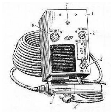
Рисунок 2.5. Индикатор-сигнализатор ДП-64:
