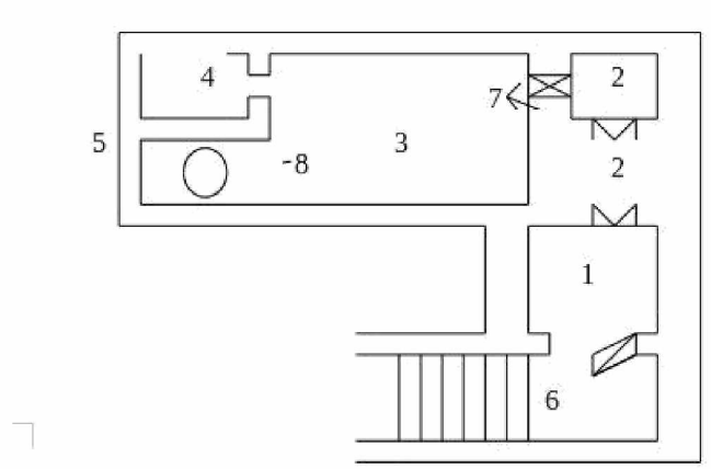
Рисунок 1.9. План типового убежища (вариант)
