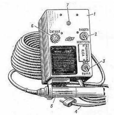
Рисунок 2.5. Индикатор-сигнализатор ДП-64:
