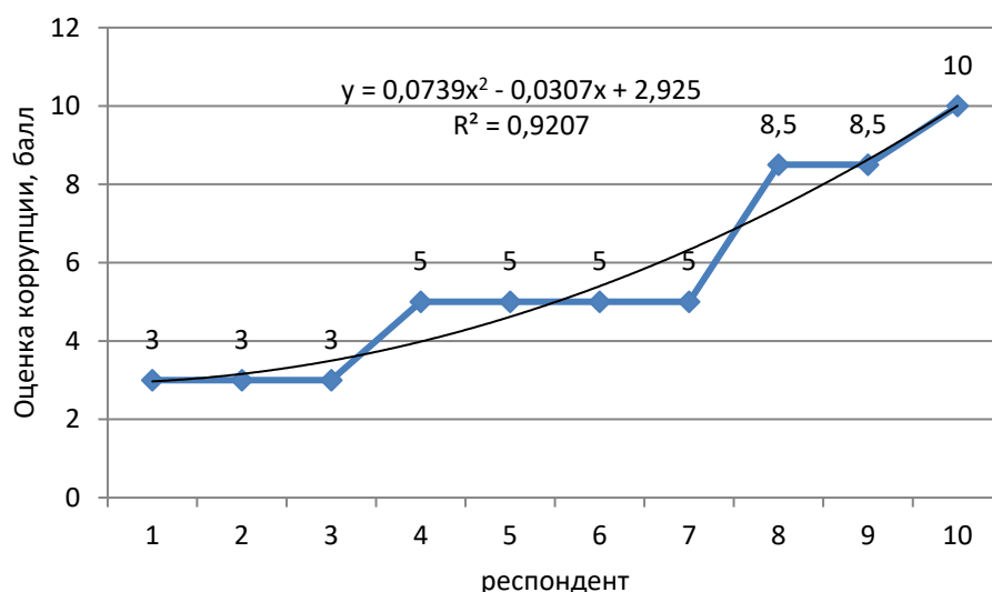
Рисунок 2 – Квадратическая полиномиальная модель изменения CPI
