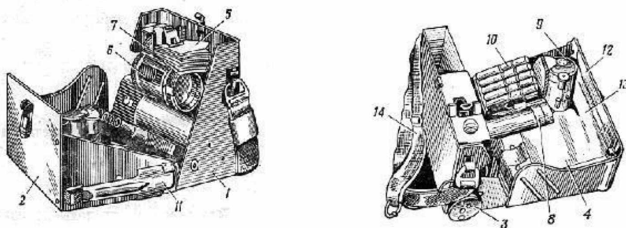
Рисунок 2.10. ВПХР: 1 — корпус; 2 — крышка; 3 — ручной насос; 4 — кассеты с индикаторными трубками; 5 — противозарозольные фильтры; 6 — насадка; 7 — защитные колпачки; 8 — фонарь; 9 — грелка; 10 — патроны к грелке; 11 — лопатка; 12 — инструкция-памятка по работе с прибором; 13 — инструкция по обнаружению фосфорорганических ОВ; 14 — плечевой ремень.
