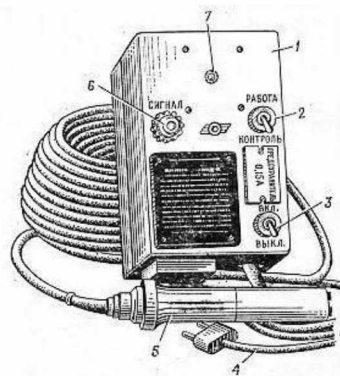
Рисунок 2.5. Индикатор-сигнализатор ДП-64:
