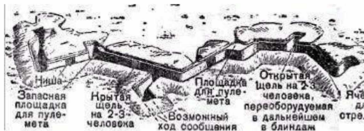
Рисунок 1.6. Окоп на стрелковое отделение
