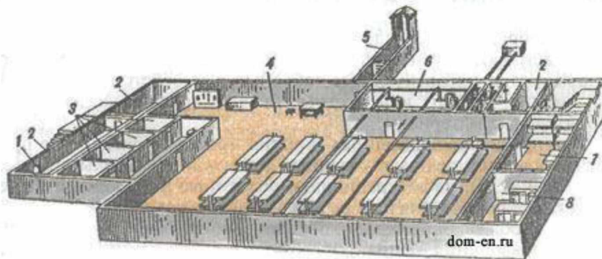
Рисунок 2.1. План убежища: 1 — защитно-герметические двери; 2 — шлюзовые камеры (тамбуры); 3 — санитарно-бытовые отсеки; 4 — основное помещение для размещения людей; 5 — галерея и оголовок аварийного выхода; 6 — фильтровентиляционная камера; 7 — кладовая для продуктов питания; 8 — медицинская комната.
