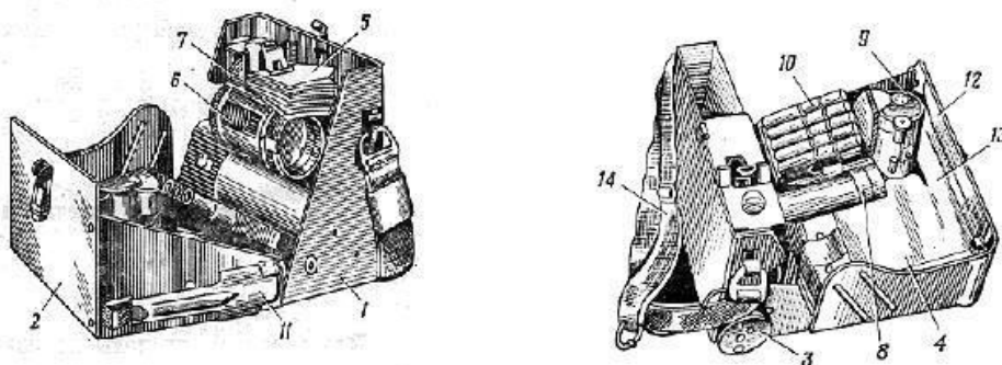
Рисунок 2.10. ВПХР: 1 — корпус; 2 — крышка; 3 — ручной насос; 4 — кассеты с индикаторными трубками; 5 — противоаэрозольные фильтры; 6 — насадка; 7 — защитные колпачки; 8 — фонарь; 9 — грелка; 10 — патроны к грелке; 11 — лопатка; 12 — инструкция-памятка по работе с прибором; 13 — инструкция по обнаружению фосфорорганических ОВ; 14 — плечевой ремень.
