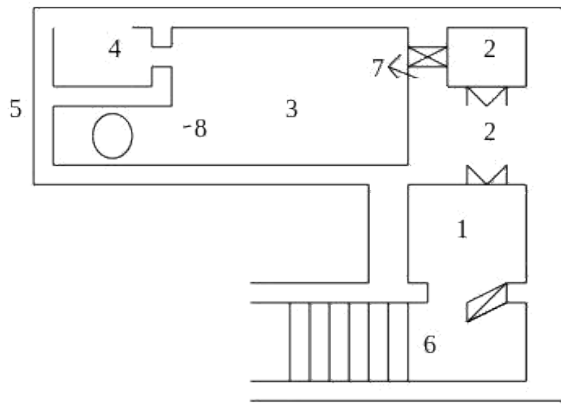
Рисунок 1.9. План типового убежища (вариант)
