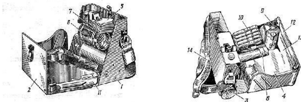
Рисунок 2.10. ВПХР: 1 — корпус; 2 — крышка; 3 — ручной насос; 4 — кассеты с индикаторными трубками; 5 — противоарозольные фильтры; 6 — насадка; 7 — защитные колпачки; 8 — фонарь; 9 — грелка; 10 — патроны к грелке; 11 — лопатка; 12 — инструкция-памятка по работе с прибором; 13 — инструкция по обнаружению фосфорорганических ОВ; 14 — плечевой ремень.
